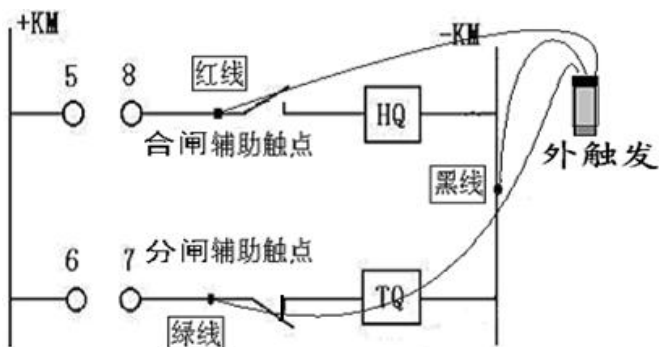
高压开关控制屏外触发控制接线示意图
